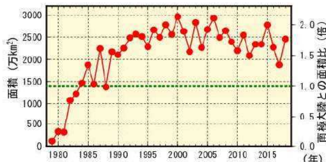
オゾンホール面積の年最大値の推移 (出典) 気象庁ホームページから
